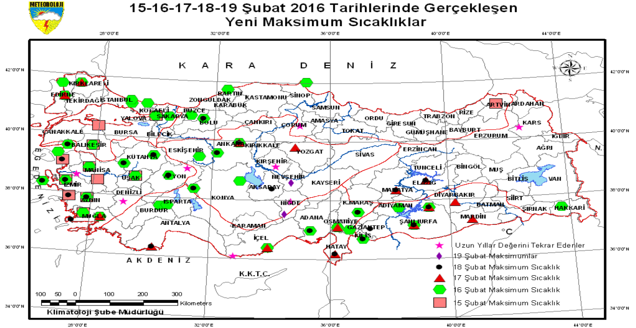
Şekil 2. 15-19 Şubat 2016 tarihleri arasında gerçekleşen aşırı sıcaklıkların dağılımı (22).
