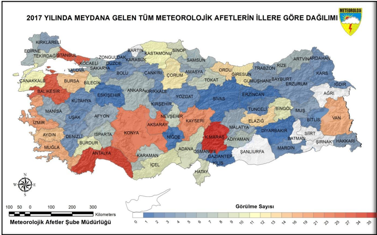
Şekil 3. Ülkemizde 2017 Yılında Meydana Gelen Meteorolojik Karakterli Doğal Afetlerin Dağılımı
