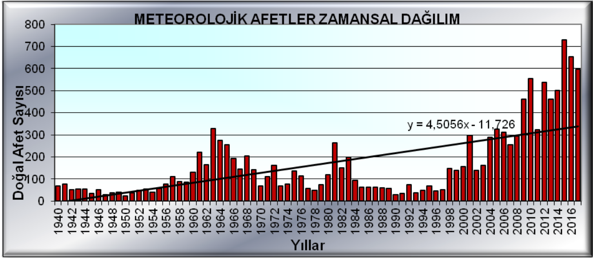
Şekil 1. Türkiye’de 1940-2017 Periyodunda Gözlenen Meteorolojik Karakterli Doğal Afetler
