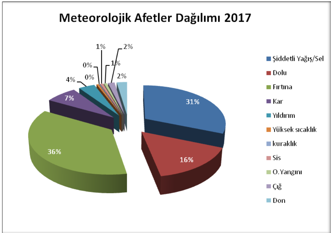
Şekil 2. 2017 Yılı Meteorolojik Karakterli Doğal Afetlerin Dağılımı
